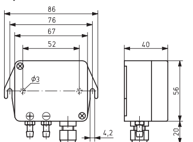
габаритный чертёж
